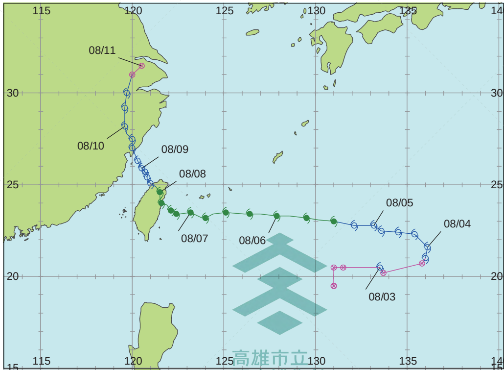
莫拉克颱風路線圖
