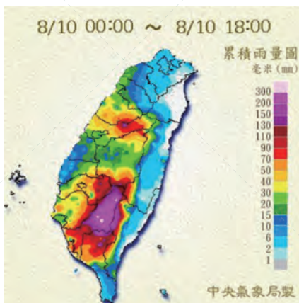
莫拉克颱風區域雨量
