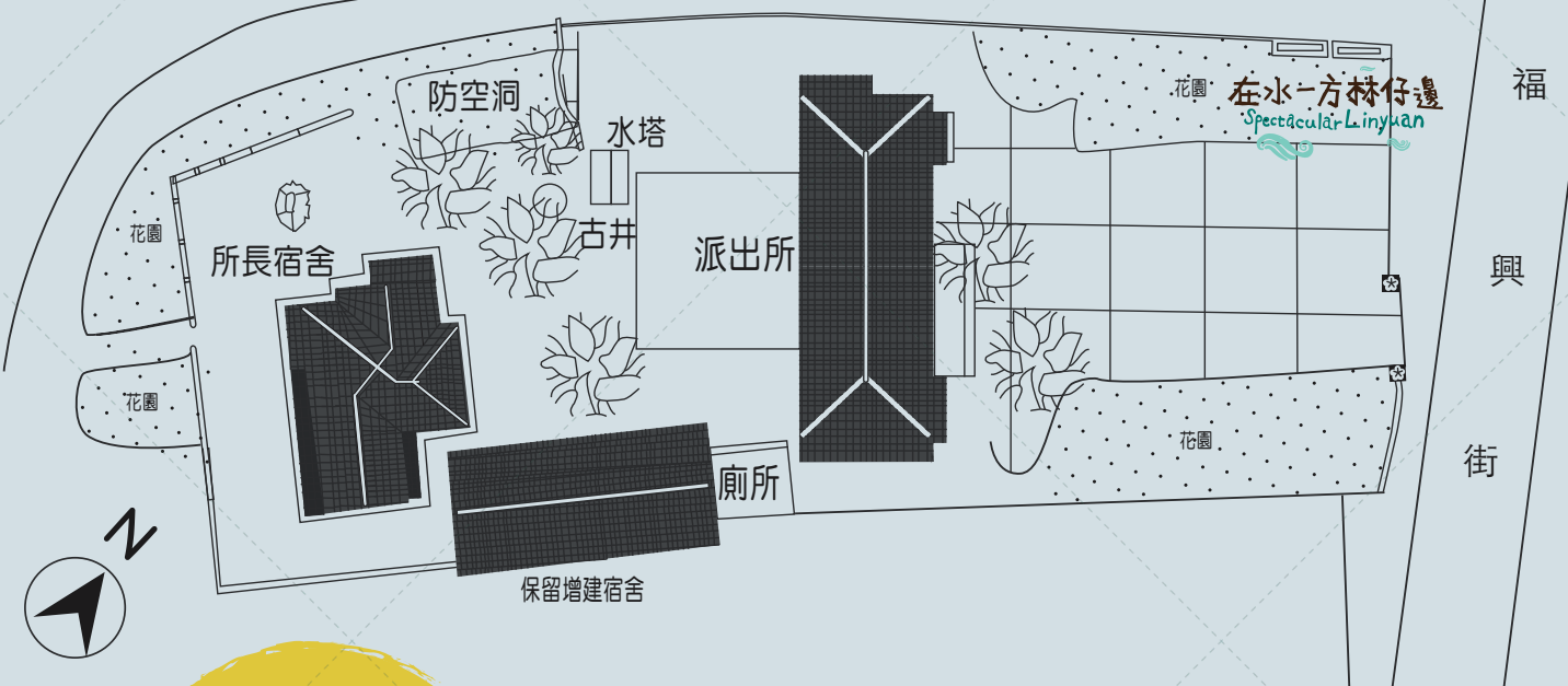
民國 101 年 (2012) 原頂林仔邊警察官吏派出所建築規模。(圖片提供：高雄市政府文化局文資中心)
