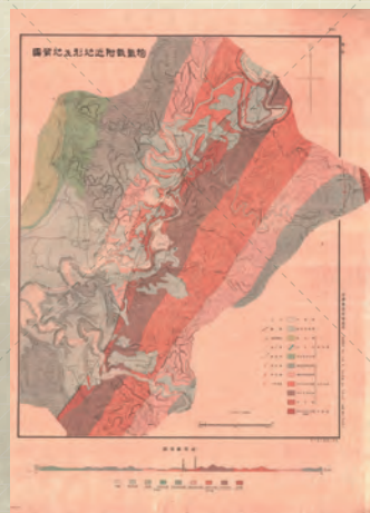
狗玢氫附近地形及地質圖。
