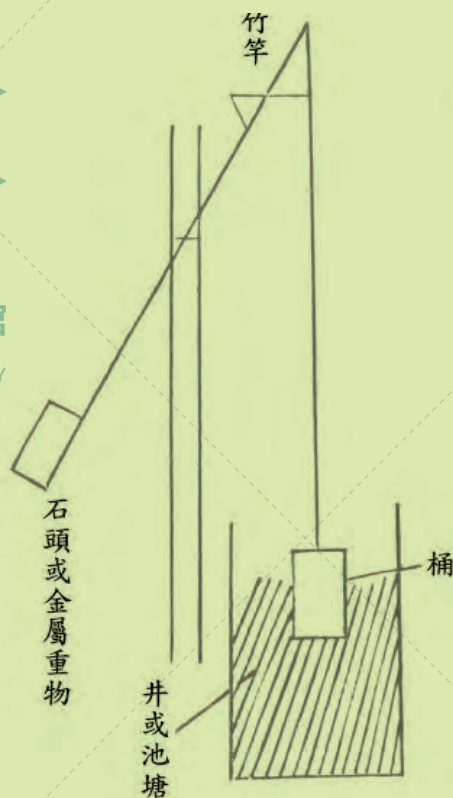
吊荷示意圖
