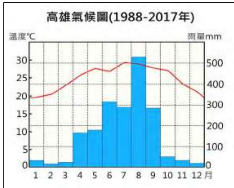
圖 2-8 西元 1988-2017 年高雄氣候圖
