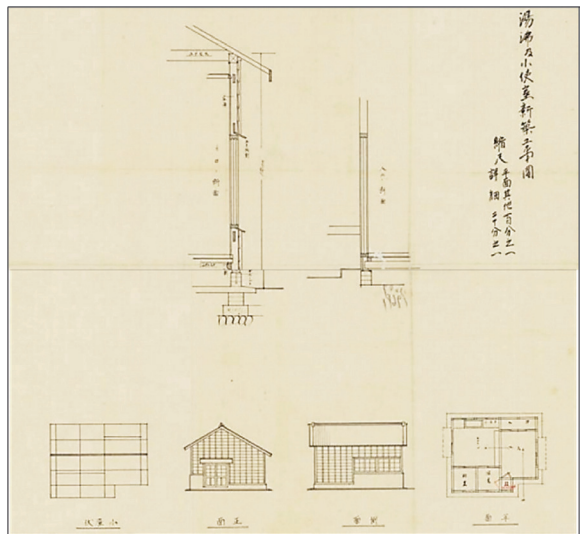
圖 2 高雄高等女學校湯沸及小使室新築工事圖
