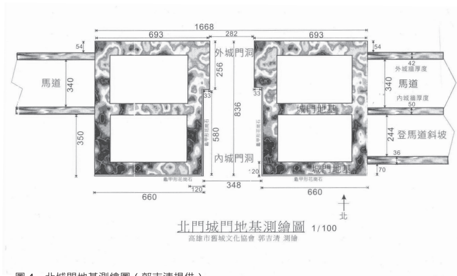
圖 4 北城門地基測繪圖 (郭吉清提供)
