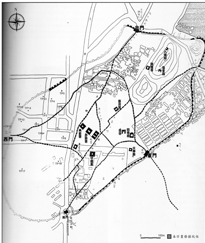
圖 5 2015 年試掘坑位套疊左營舊城城內空間圖（底圖取自李乾朗《鳳山縣舊城調查研究》，頁 55）
