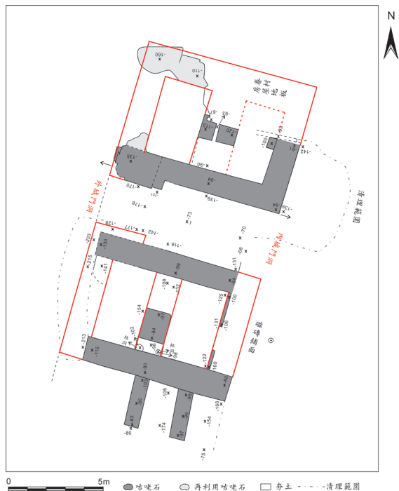
圖 3 西城門基礎保存狀況與復原圖
